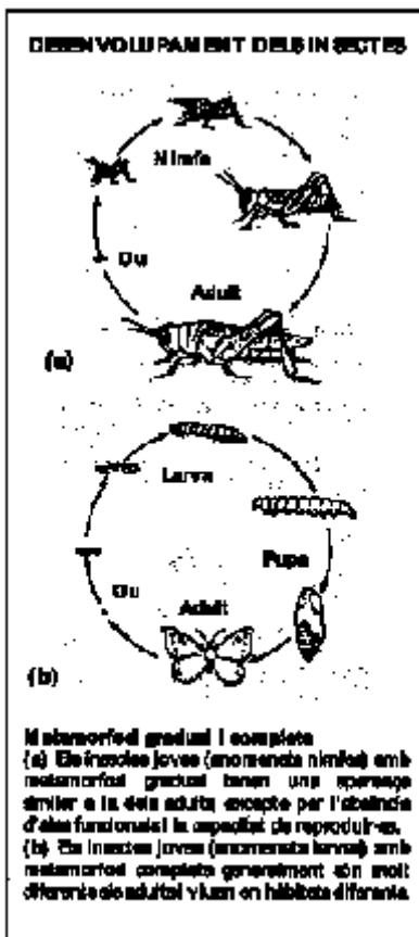
Fig. 3.2.- Desenvolupament dels insectes amb metamorfosi.
