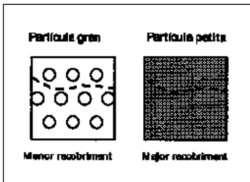
Fig. 3.7- Si es representa en un dibuix esquemàtic dues superfícies a les quals s'ha fet una aplicació homogènia amb una mida de partícula diferent, el que es veu és que en la trajectòria d'un individu podria no haver-hi contacte amb el plaguicida si la partícula és gran.
